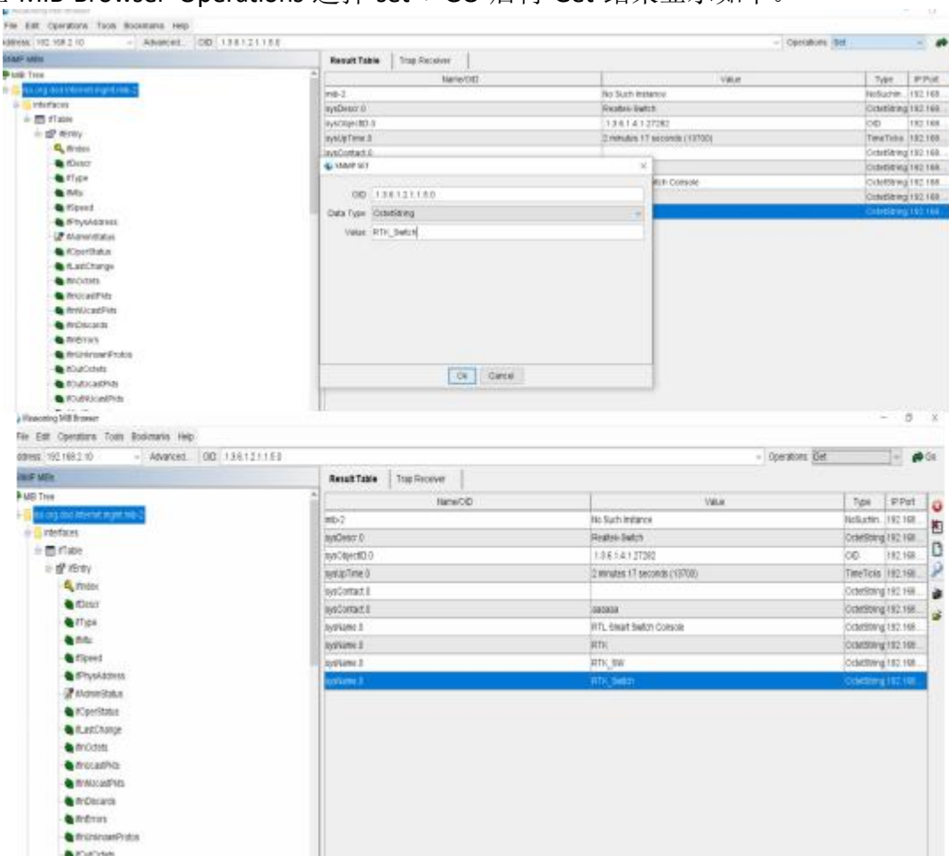
图 74 SNMP Trap Set
